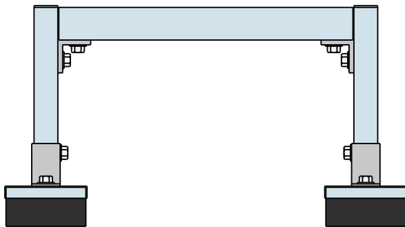
Elevation
