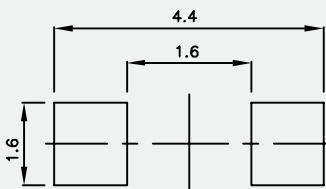
KPL-3015
