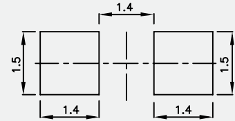
KA-3021
