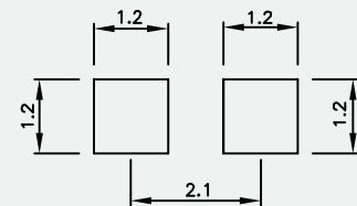
KPHCM-2012
