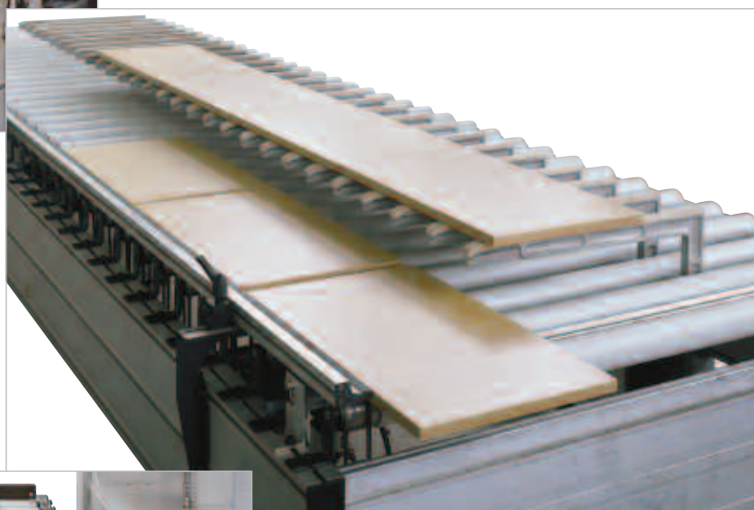
Transfer con sistema a pettine per carico pannelli in doppia fila.
