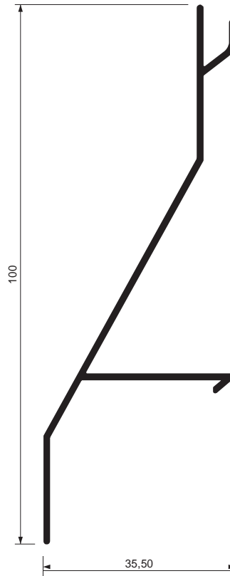
050020 LAMA Z Escala 1:1 Scale 1:1 Echelle 1:1 SLAT Z LAME Z
