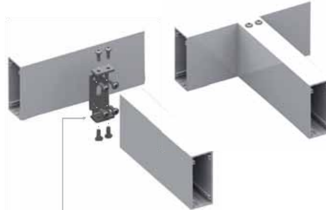
023113 PIEZA DE UNIÓN FRONTAL PERFIL PORTANTE UNION FRONT PIECE SUPPORT PROFILE PIÈCE D'UNION FRONTALE PROFIL SUPPORT
