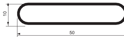
050160 LAMA D-5 Escala Scale 1:1 SLAT D-5 Échelle LAME D-5
