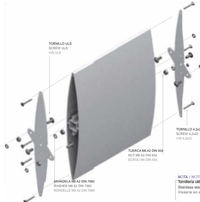
POSICIONES TESTEROS SISTEMA FIJO / POSITIONS FIXED END CAPS /
