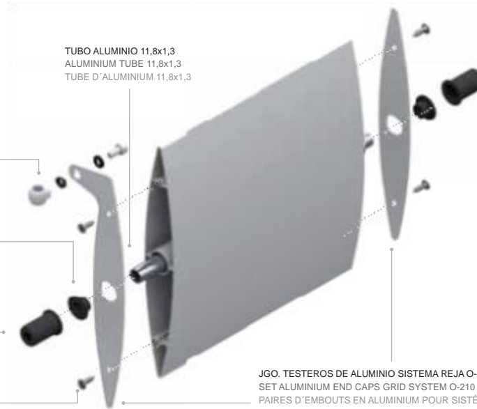
JGO. TESTEROS DE ALUMINIO SISTEMA REJA SET ALUMINIUM END CAPS GRID SYSTEM PAIRES D'EMBOUITS EN ALUMINIUM POUR SYSTÈME GRILLE
