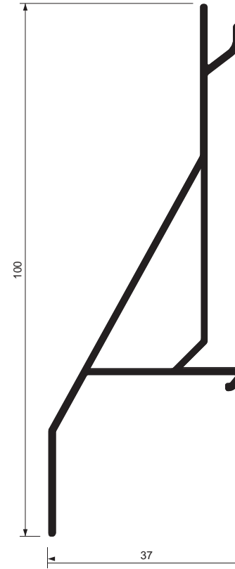
050001 LAMA Z / PVC Escala 1:1 Scale 1:1 Echelle 1:1 SLAT Z / PVC LAME Z / PVC
