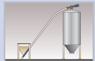
Loading silos.
