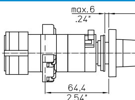
S0 Q120/A1 - S0 Q120/A5 Q120 Push-to-turn operation with a/c C-, DH-switches
