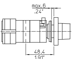
S0 Q120/A1 - S0 Q120/Z00Z5 Q120 Push-to-turn operation without a/c C-, DH-, DK-switches
