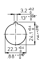
S0 Q120/A1 - S0 Q120/A5 Q120 Push-to-turn operation with a/c C-, DH-switches
