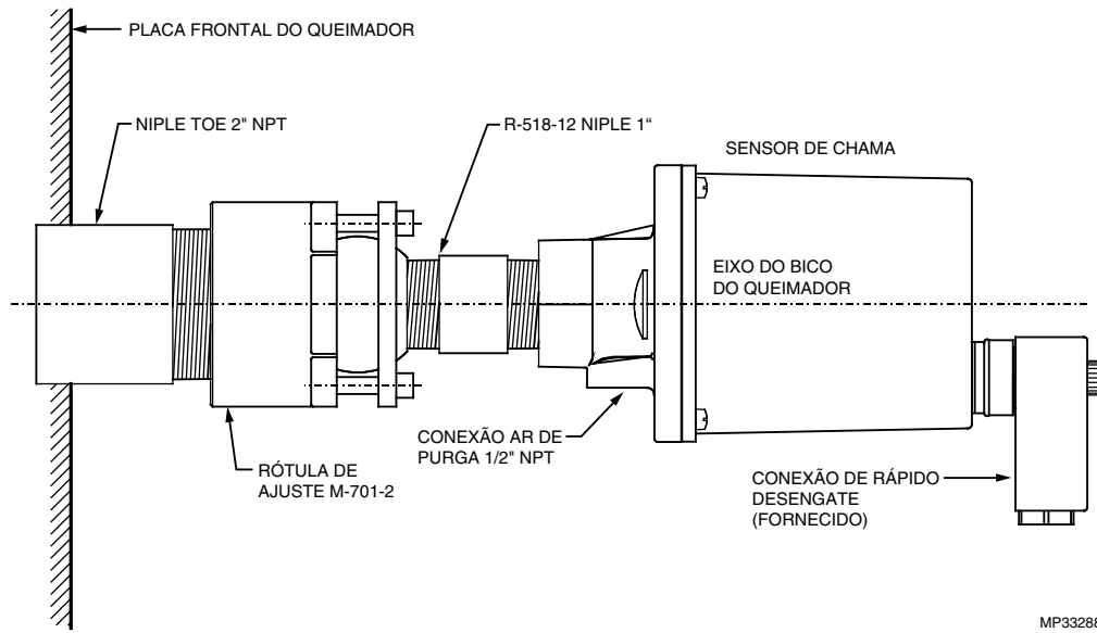
Fig. 7. Exemplo de montagem do sensor de chama.
