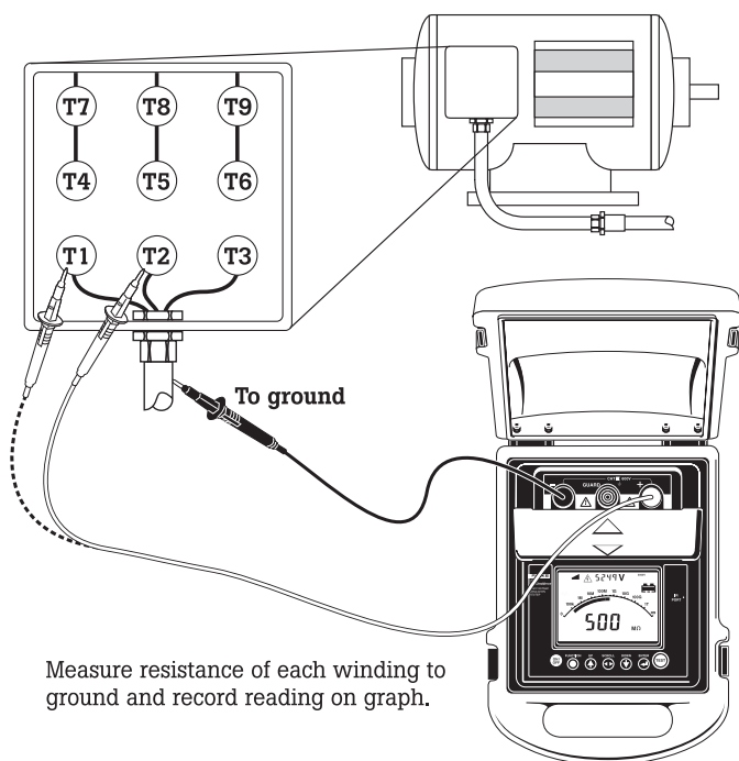
Megohmmeter
