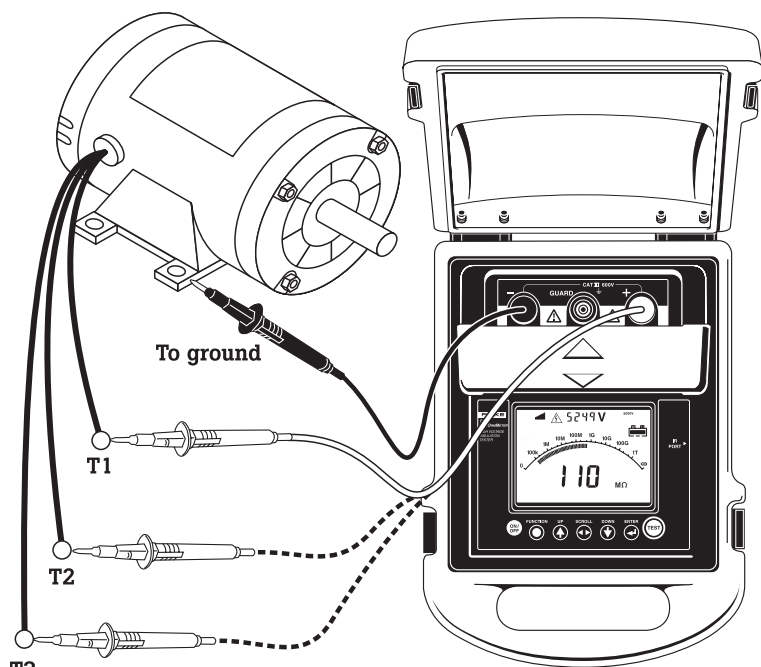
Megohmmeter
