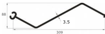
Z rib
