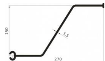
DuoRib
