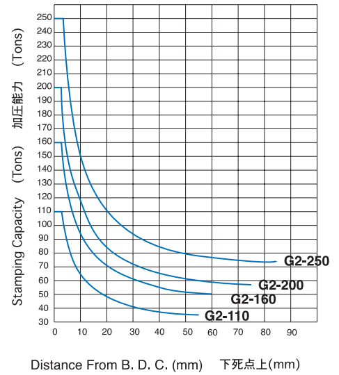
Stroke-Capacity Diagram ( H ) ストローク/能力曲線図(H)
